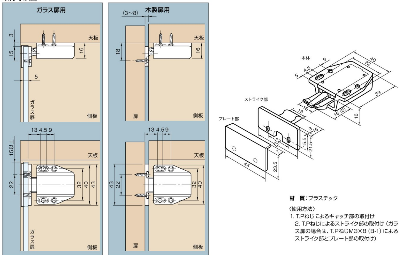
取付寸法図
