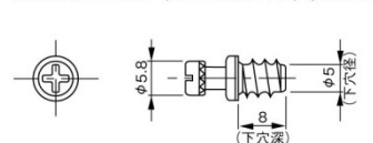
システム7-シャフト (スクリュウタイプ) \phi 5 \times 7.5 (MT06402ZN)
