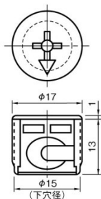
エキセンティージョイント 本体
