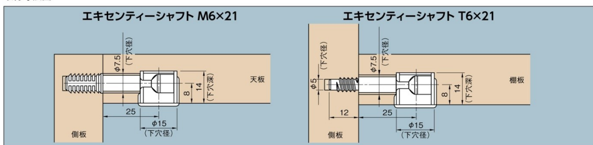
取付寸法図
