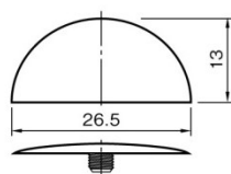
タイトスキャップA
