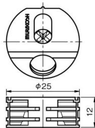
タイトスジョイント
