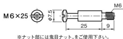
固定ピン
