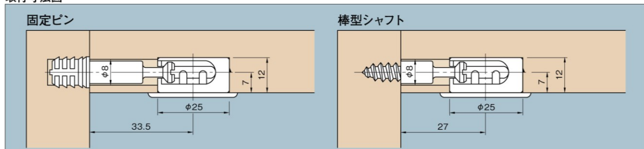
取付寸法図
