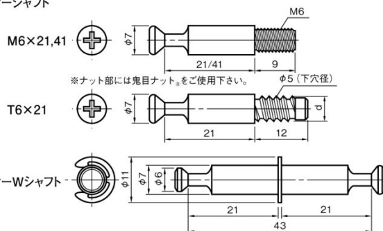
エキセンティーシャフト
