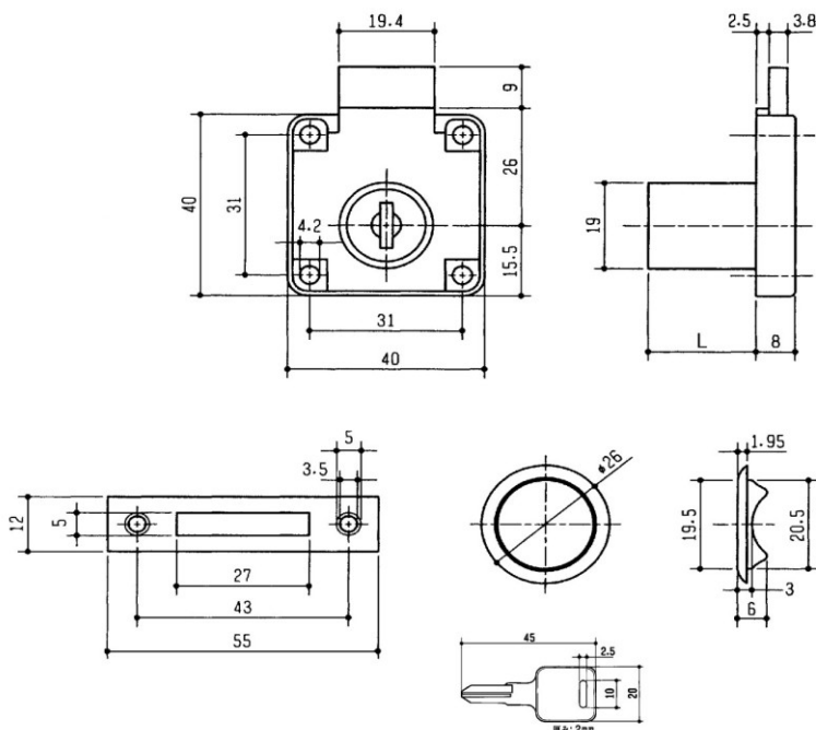
507-26 戸厚26mm用
