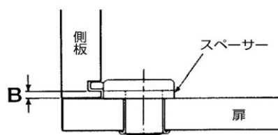
右開きかぶせ扉へのスペーサー取付例
