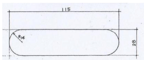
取付け穴参考寸法
