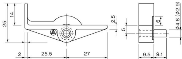
差込み棚ダボTM
