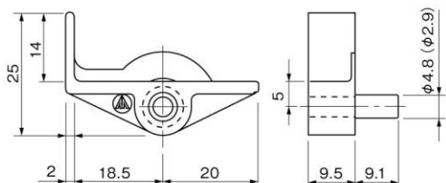
差込み棚ダボGM
