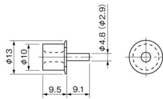
差込み棚ダボM
