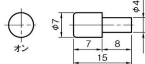
差し込みB
