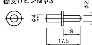
棚受けピンMφ3
